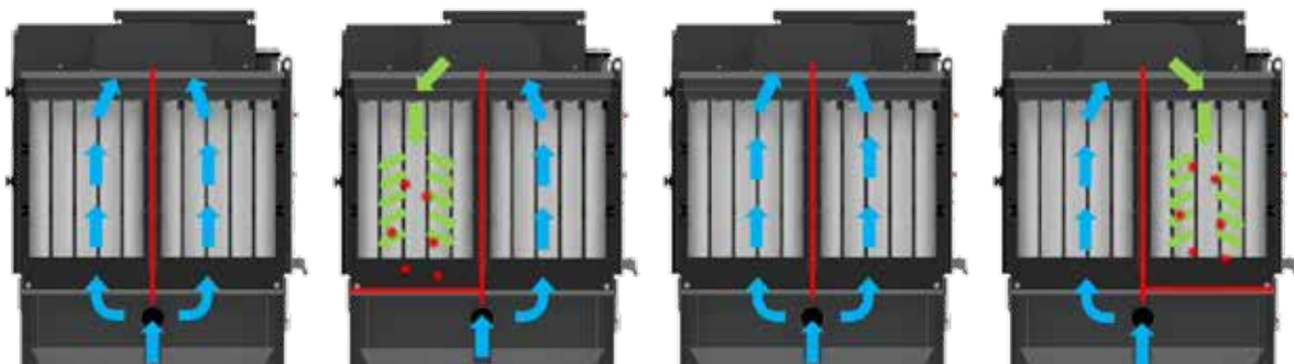
Werkingsprincipe van het filterreinigingssysteem Filter cleaning system operating principle
